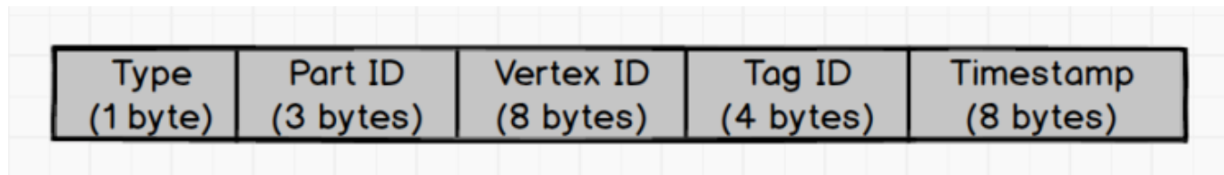
图二 Vertex Key Format
