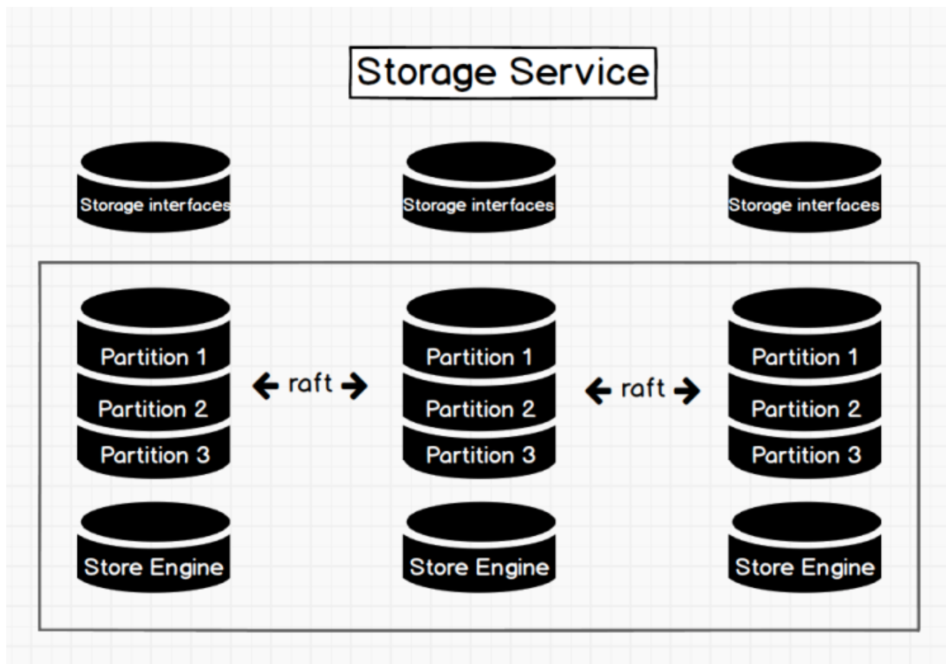
图一 storage service 架构图
